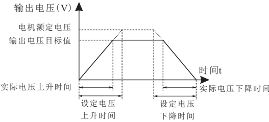
图6-8 V/F分离示意图
