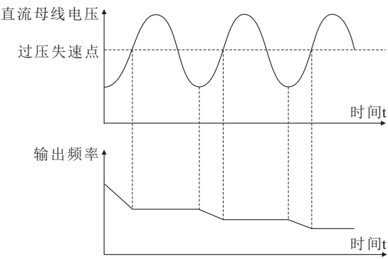
图6-10 过压失速功能
