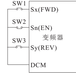
图6-14 三线式运转模式1
