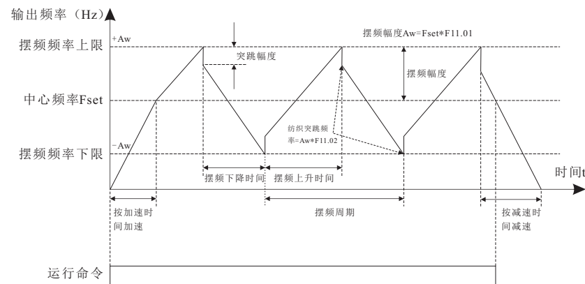
图6-32 摆频工作示意图
