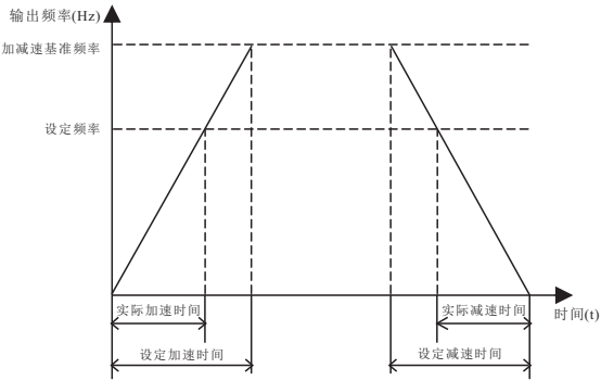
图6-1 加减速时间示意图
