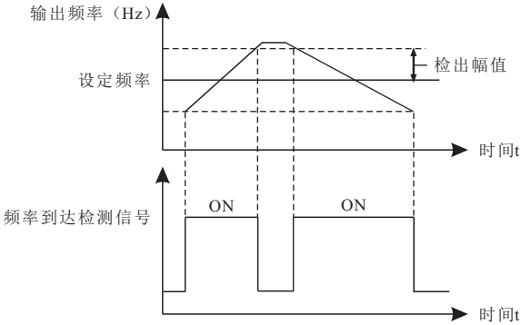
图6-21 频率到达检出幅值示意图
