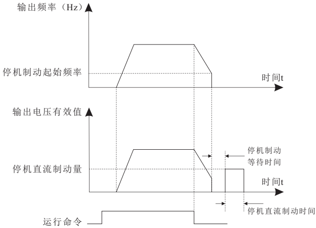
图6-4 停机直流制动示意图
