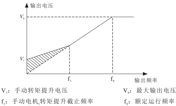
图6-6 手动转矩提升示意图
