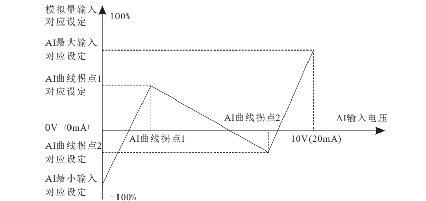
图6-17 曲线4和曲线5示意图
