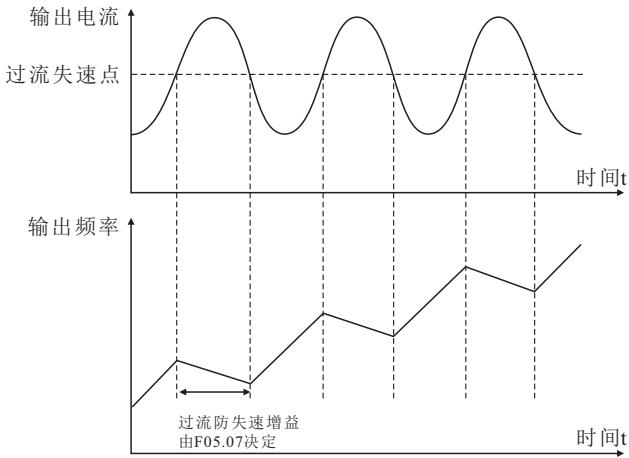
图6-11 过流防失速保护功能示意图
