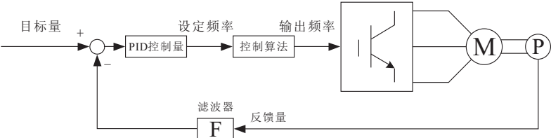
图6-28 过程PID原理框图
