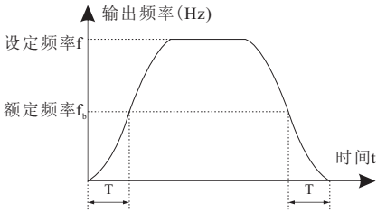
图6-3 S曲线加减速B示意图
