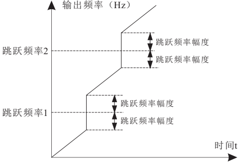
图6-22 加减速过程中跳跃频率有效示意图
