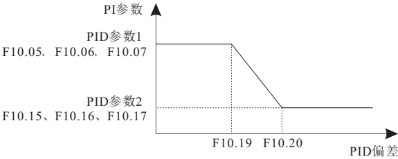
图6-30 PID参数切换
