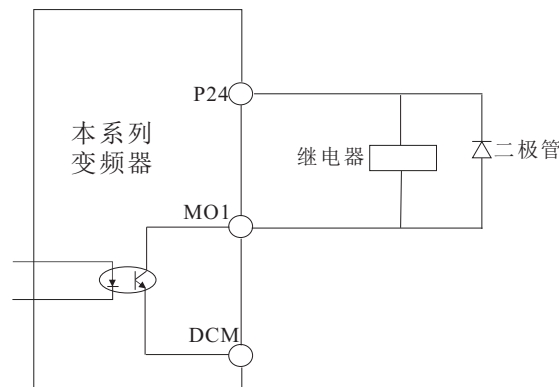
图3-7 数字输出端子接线示意图
