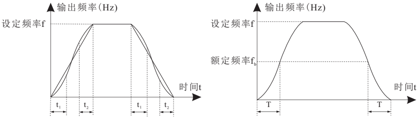
图6-2 S曲线加减速A示意图
