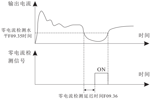
图6-25 零电流检测示意图
