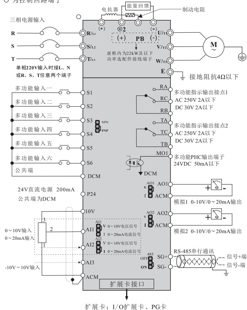
图3-3 基本配线图
