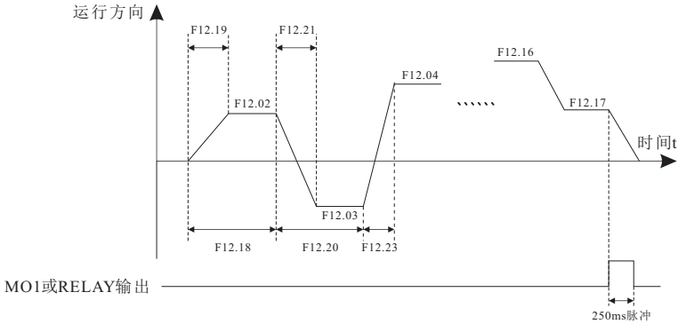
图6-34 简易PLC示意图
