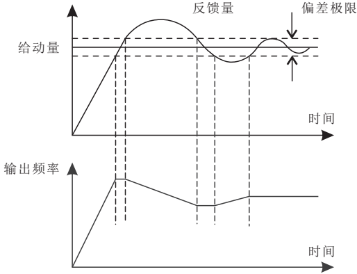
图6-29 偏差极限与输出频率的对应关系
