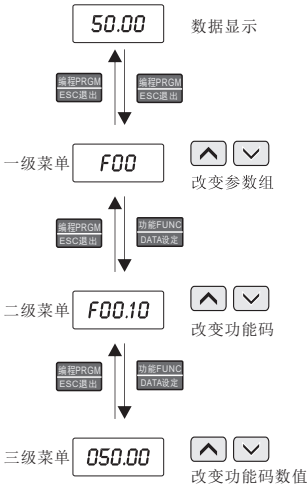
图4-2 三级菜单操作流程图
