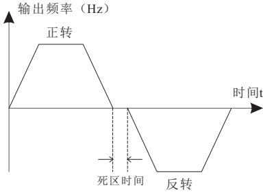
图6-19 正反转死区时间示意图
